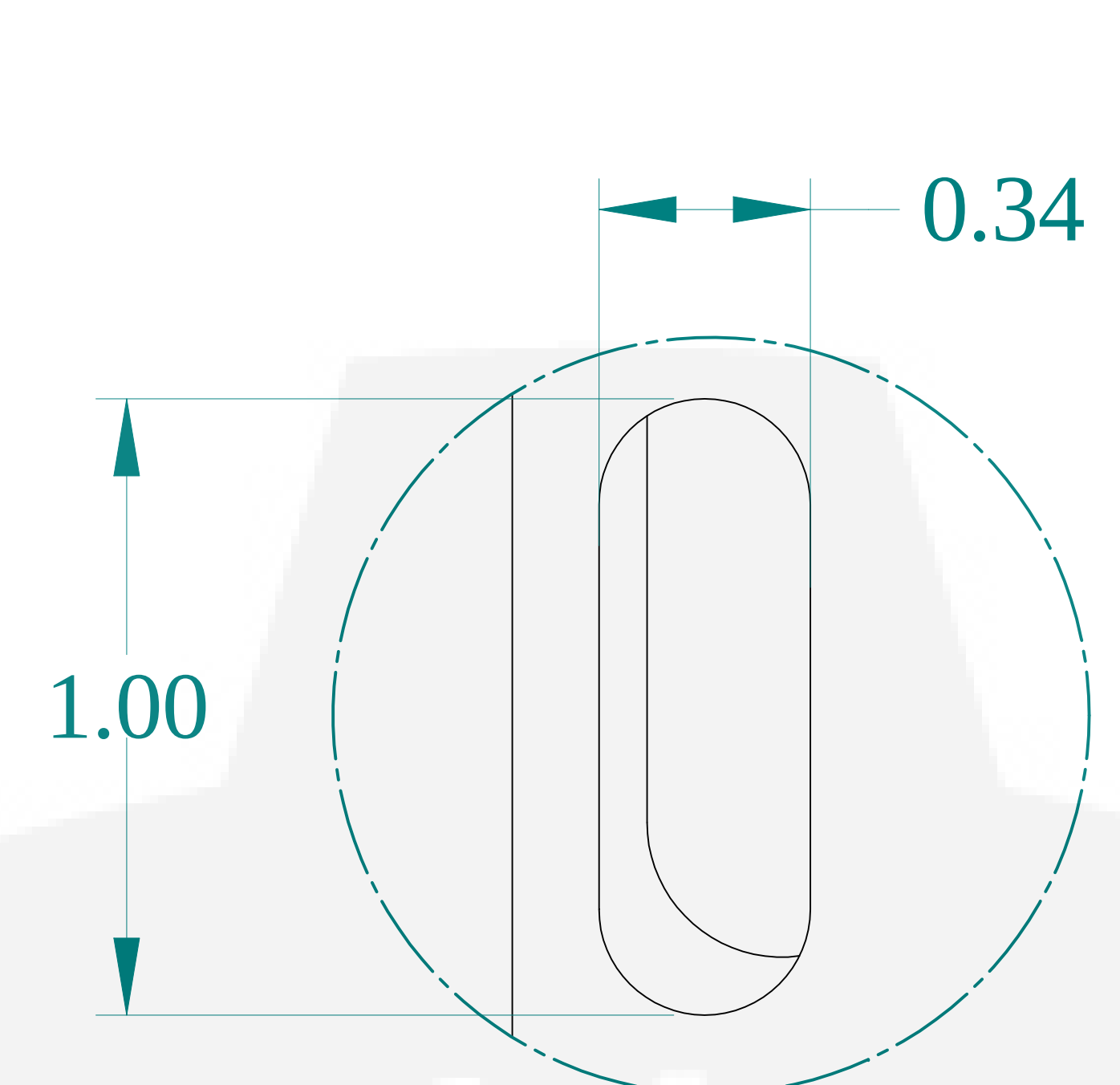
DETAIL Z TYP
