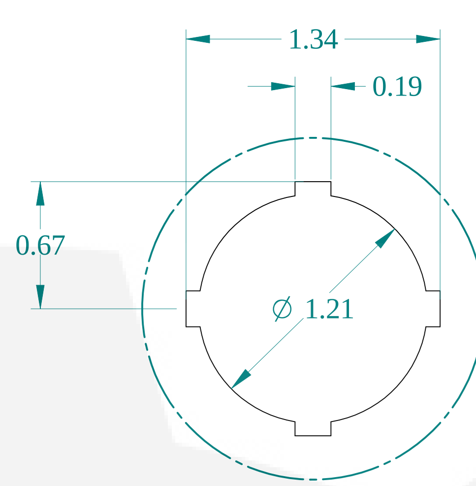
DETAIL Y
