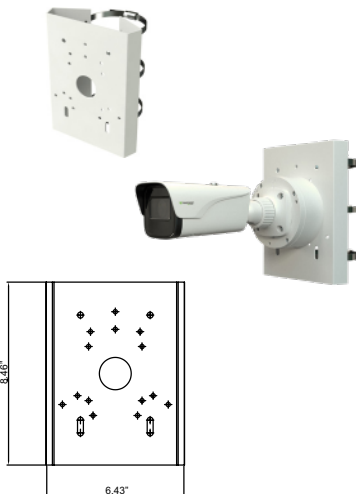
VT-TPLMT Transcendent Universal Pole Mount (reqs. VT-TJB08)
