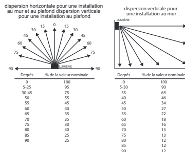
POURCENTAGE DE L'INTENSITÉ LUMINEUSE MESURÉE DANS LES DIRECTIONS SUIVANTES – SELON LA NORME UL 1971
