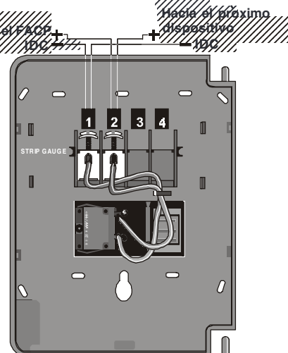
Alambrado de la BG-12, 12L, 12LSP de Acción Doble
