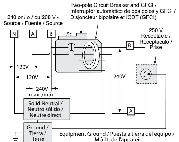
FIG. 3 : Two-wire 240 V or 208 V Circuits / Circuitos de 2 hilos de 240 V~ o 208 V~ / Circuits à 2 fils de 240 V ou 208 V
