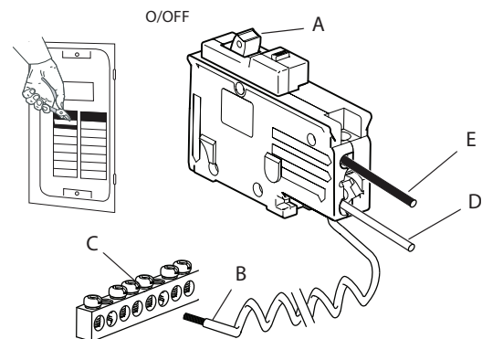
FIG. 1 : Installation / Instalación / Installation
