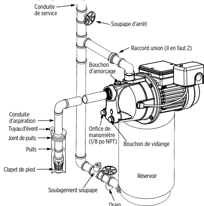
Puits peu profond système de réservoir monté
