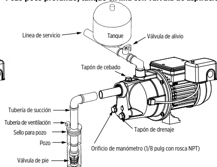
Pozo poco profundo, tanque en línea con válvula de aspiración
