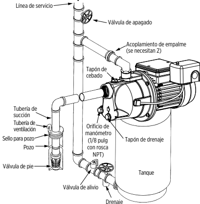
Pozo poco profundo, sistema montado en tanque con válvula de aspiración
