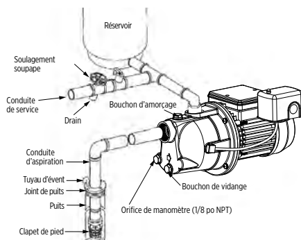
Puits peu profond avec clapet de pied
