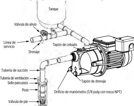
Pozo poco profundo, sistema montado en tanque con válvula de aspiración
