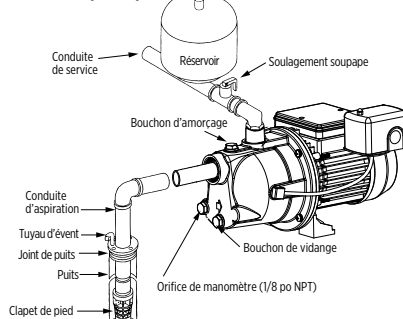
Puits peu profond, réservoir en ligne avec clapet de pied
