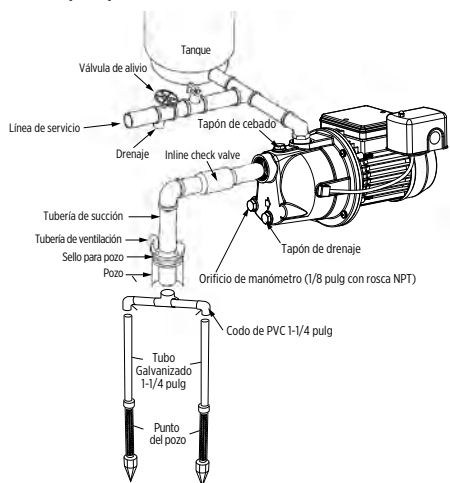
Pozo poco profundo con válvula de retención en línea
