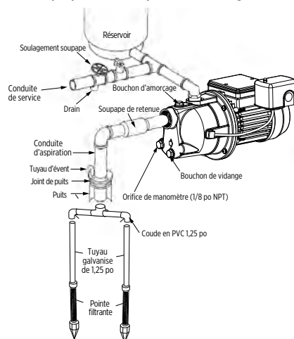
Puits peu profond avec clapet anti-retour en ligne
