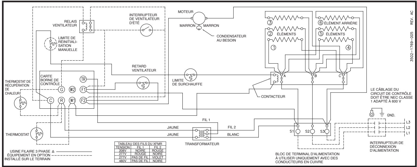
Diagramme 5: 6 éléments, 3 phases (des modèles 2YU72, 2YU73, 2YU75 et 2YU76)
