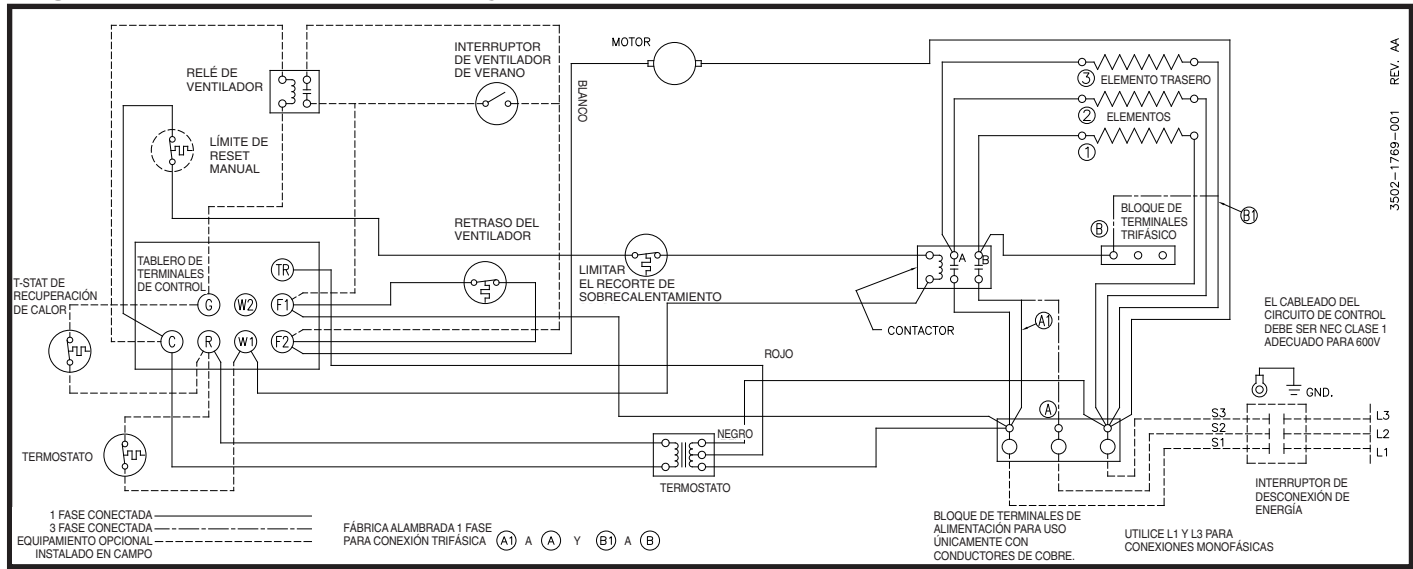
Diagrama 1: 3 elementos, monofásico y trifásico
