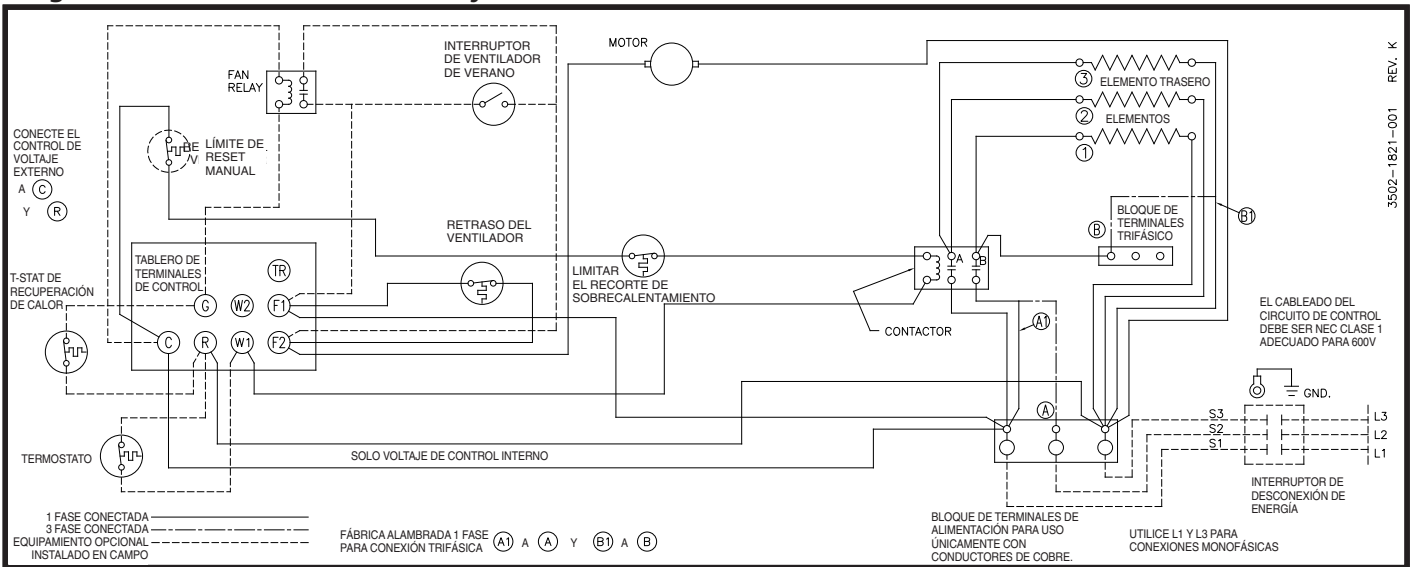
Diagram 4: 3 elementos, monofásico y trifásico
