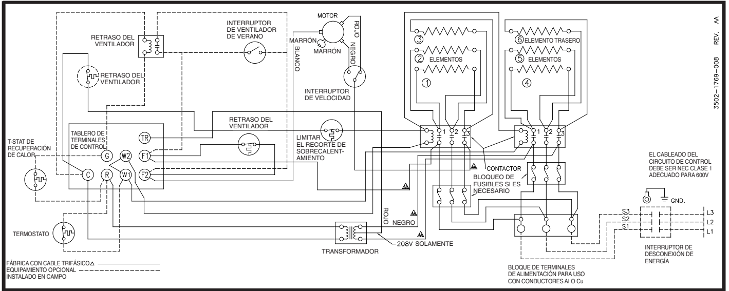
Diagram 7: 6 elementos, 2 contratista, trifásico
