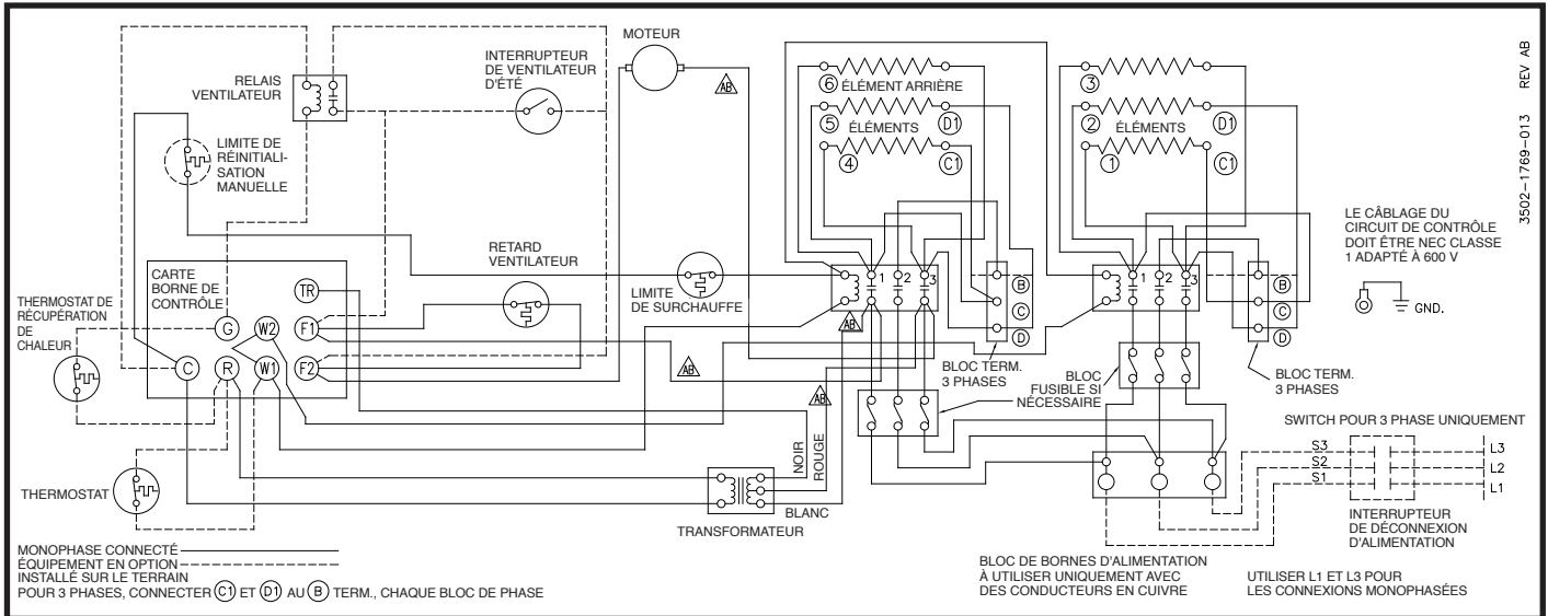
Diagramme 10: 6 éléments, monophasé et triphasé (des modèles 3END3 et 2YU78)
