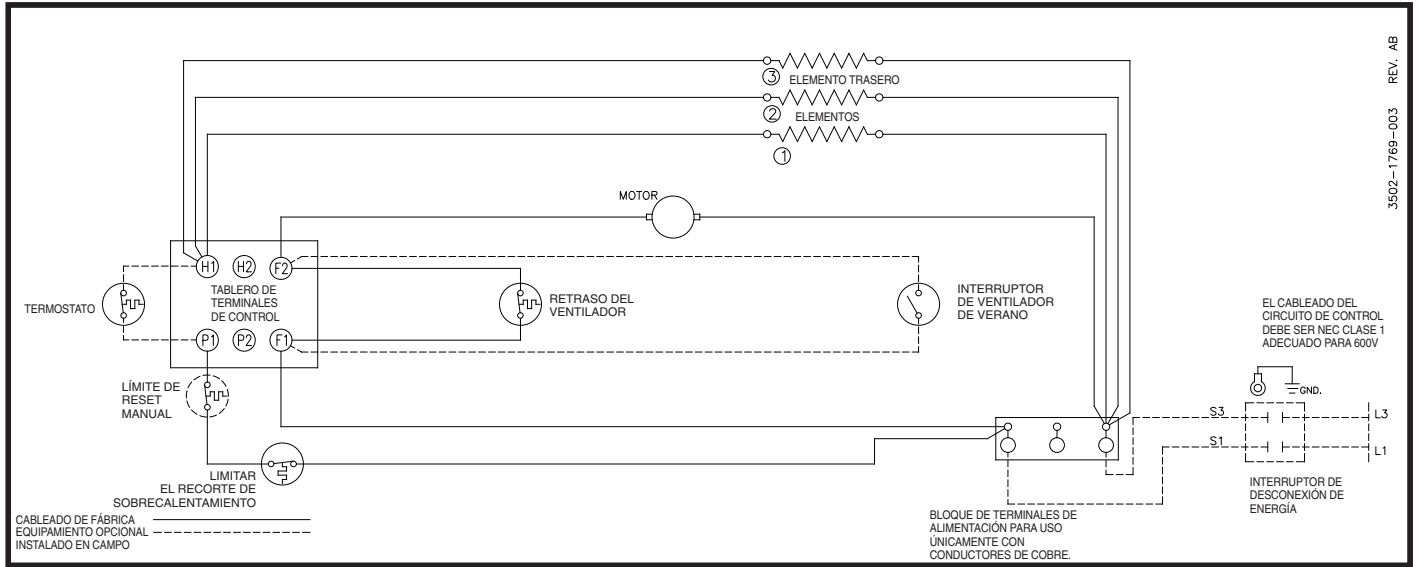
Diagram 3: 3 elementos, monofásico
