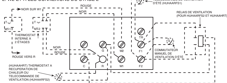
Figure 5. Carte de terminaison de commandes (pour radiateurs avec contacteur)
