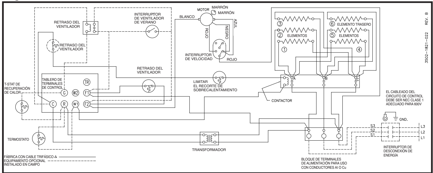
Diagram 6: 6 elementos, trifásico
