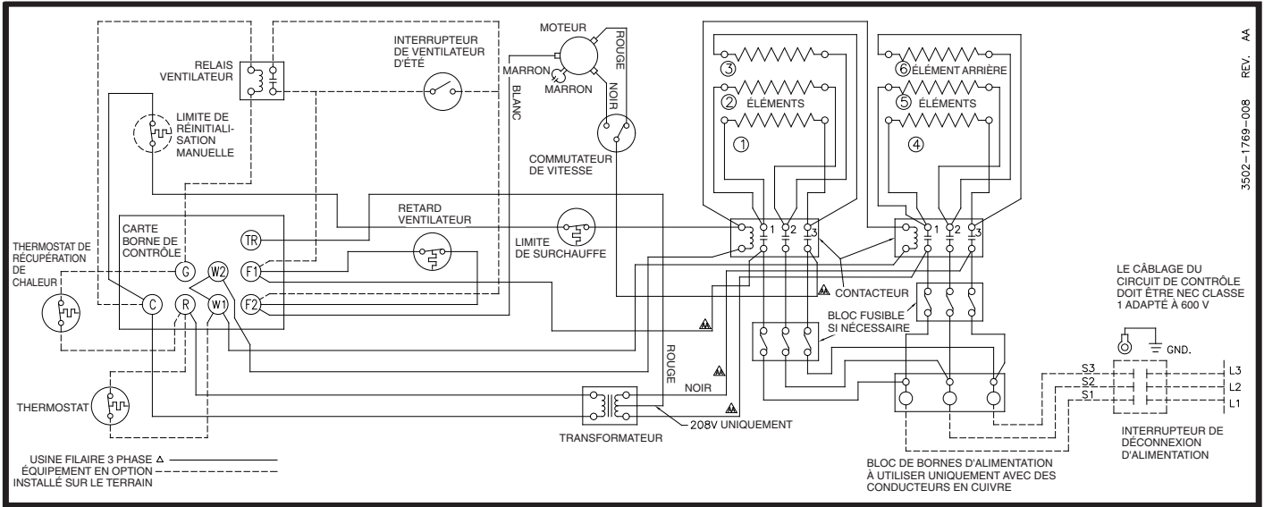
Diagramme 7: 6 éléments, 2 entrepreneurs, 3 phases (modèle 2YU77)
