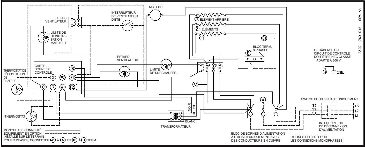
Diagramme 11: 3 éléments, monophasé et triphasé (modèle 2YU71)
