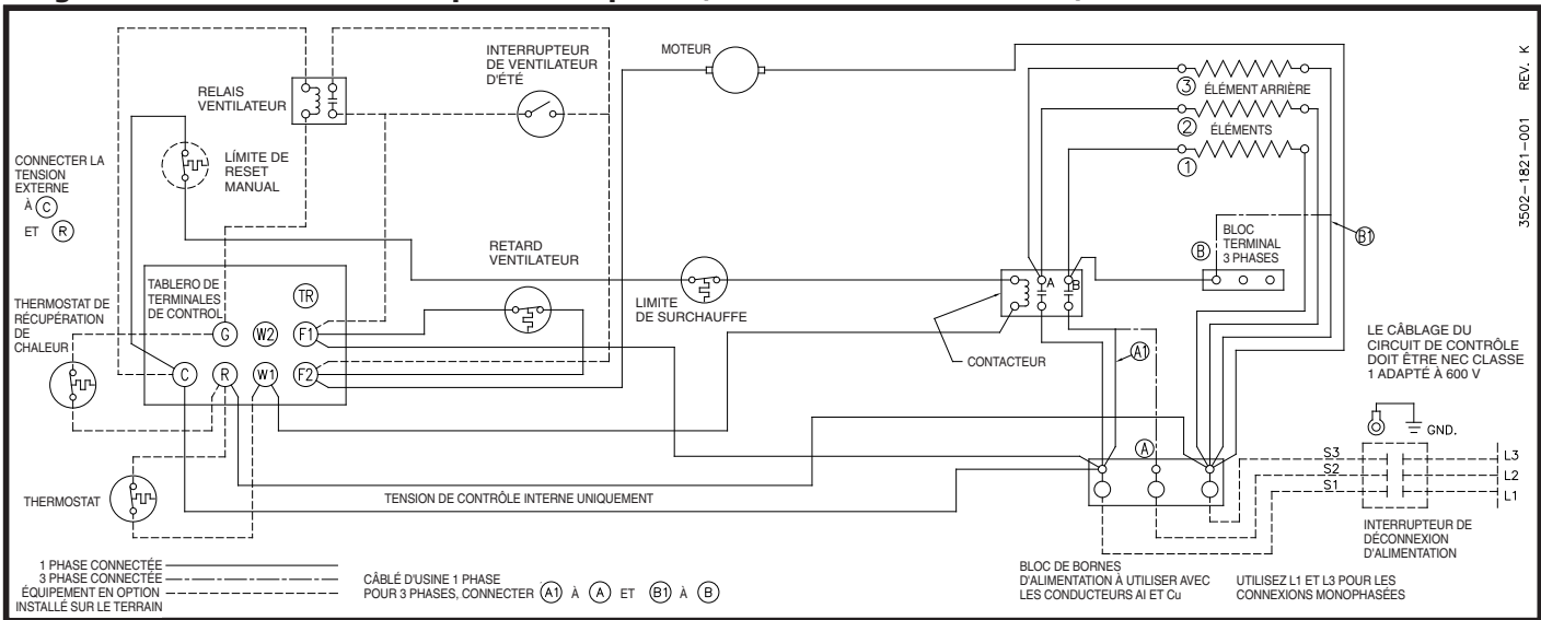
Diagramme 4: 3 éléments, monophasé et triphasé (des modèles 2YU62, 2YU65)
