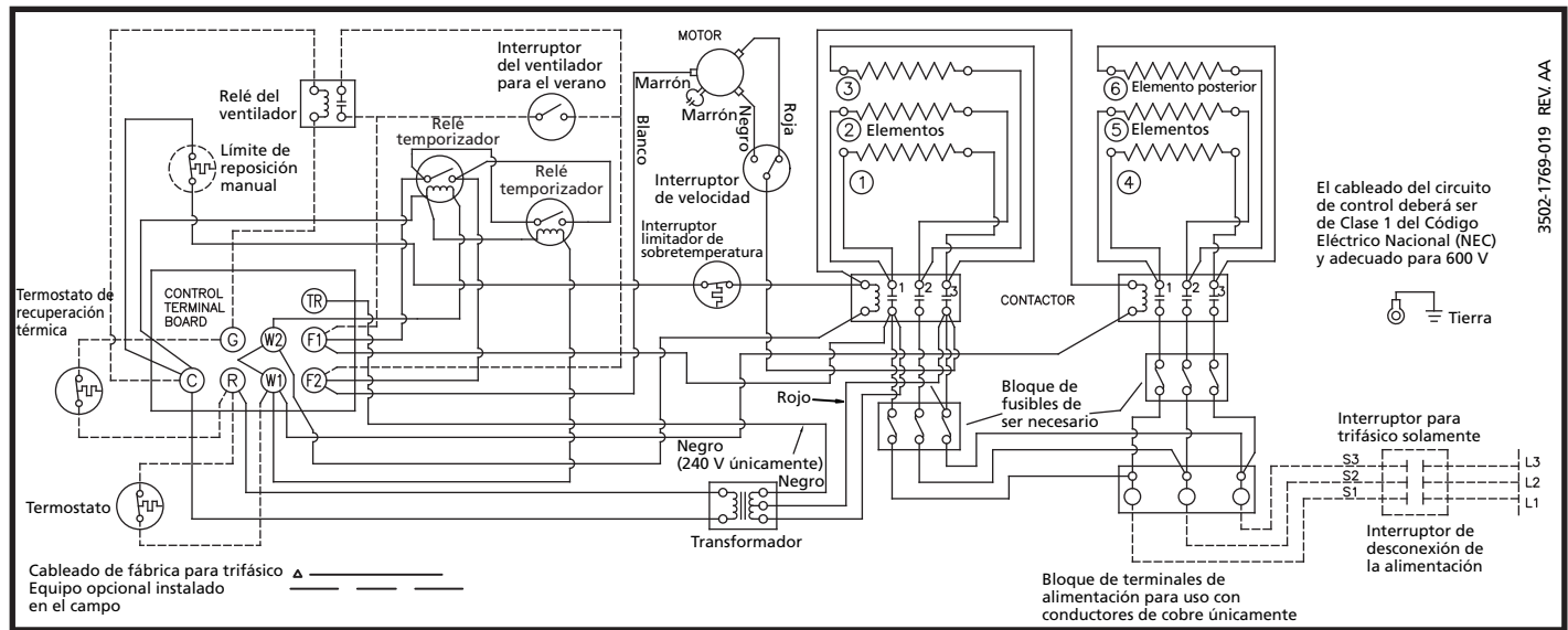
Diagrama 13: 6 Elementos, 2 Contactores, Trifásicos
