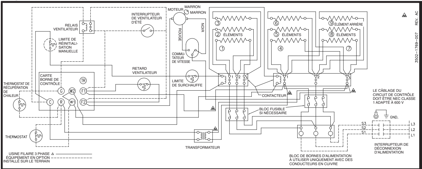
Diagramme 8: 9 éléments, 2 entrepreneurs, 3 phases (des modèles 3END4 et 2YU81)
