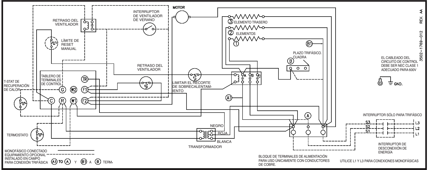
Diagrama 11: 3 elementos, monofásico y trifásico
