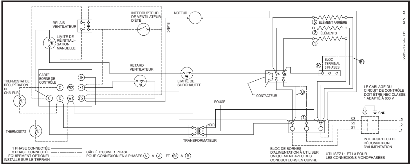
Diagramme 1: 3 éléments, monophasé et triphasé (des modèles 2YU66 et 2YU69)
