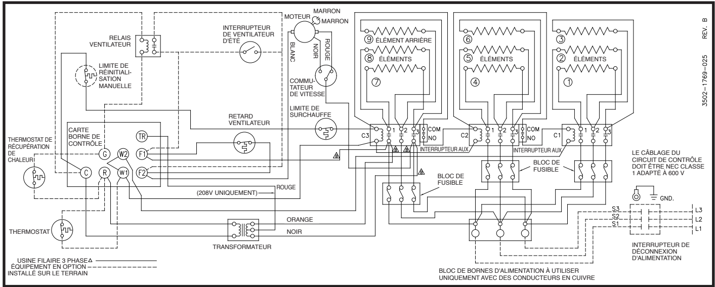
Diagramme 9: 9 éléments, 3 entrepreneurs, 3 phases (modèle 2YU80)
