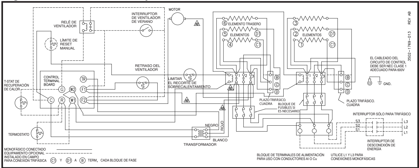
Diagrama 10: 6 elementos, monofásico y trifásico
