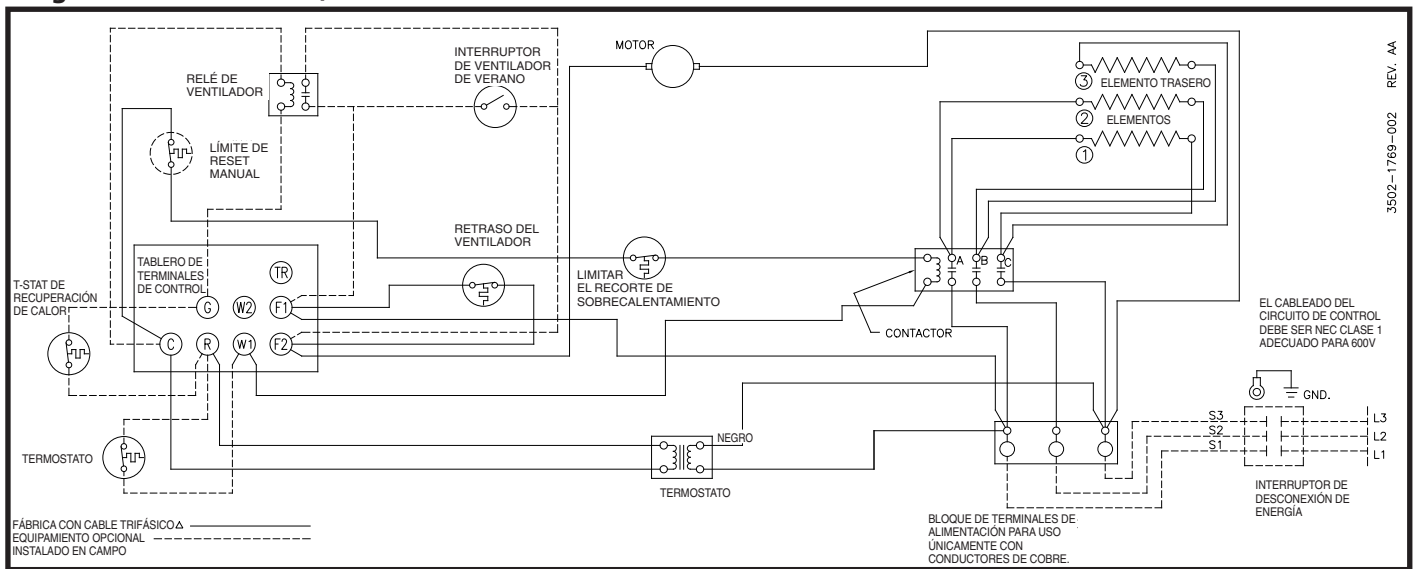
Diagrama 2: 3 elementos, trifásico
