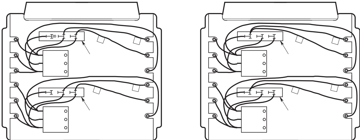
Figure 3a. Raccordements d’alimentation pour du secteur monophasé et triphasé (MUH0521, MUH0581, MUH072, MUH078, MUH102 et MUH108)
