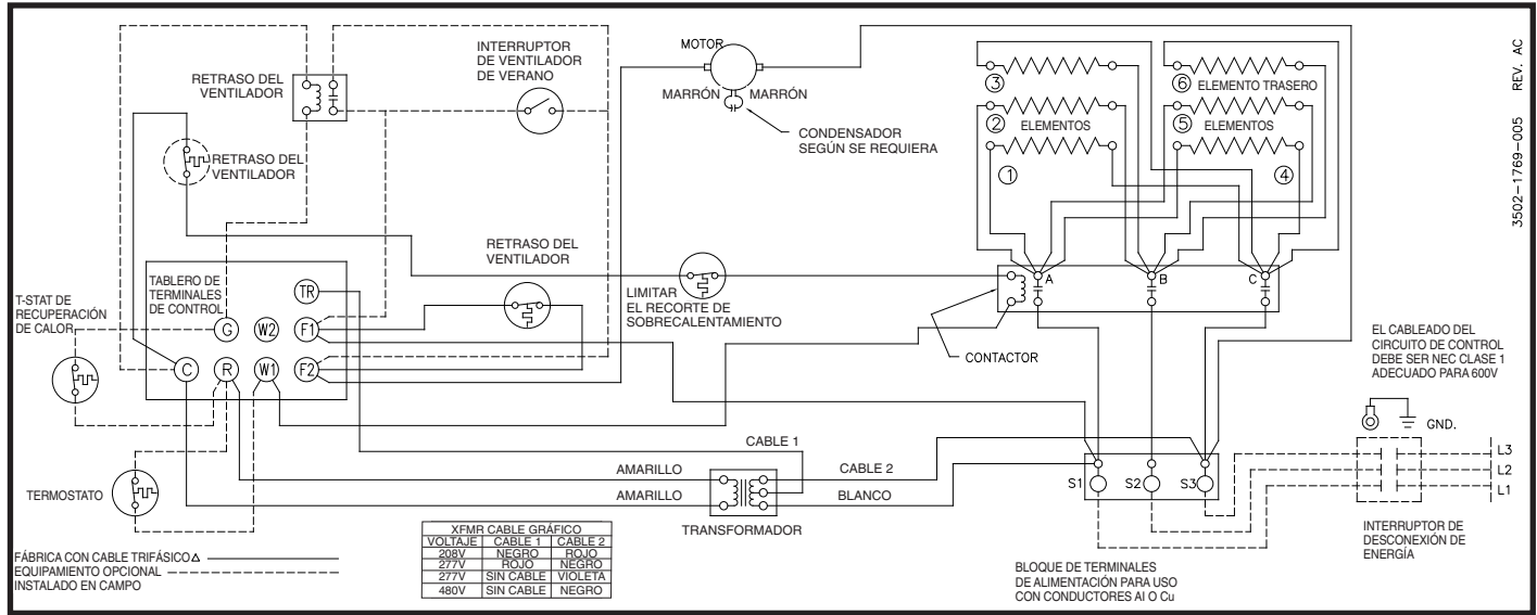
Diagram 5: 6 elementos, trifásico
