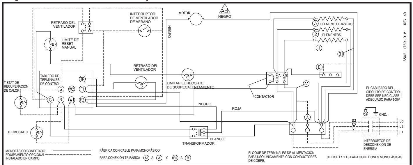
Diagrama 12: 3 elementos, monofásico y trifásico
