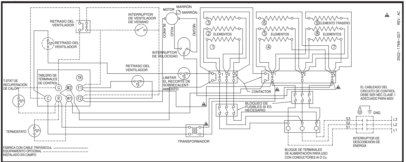
Diagram 8: 9 elementos, 2 contratistas, trifásicos
