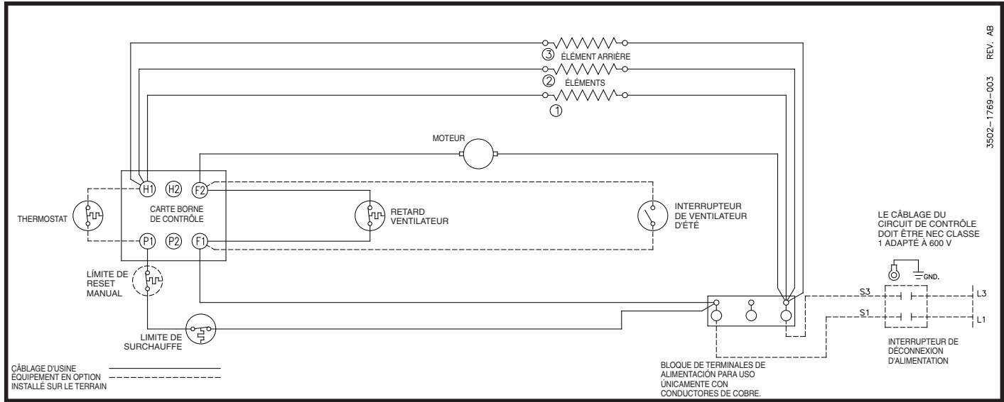
Diagramme 3: 3 éléments, monophasé (des modèles 2YU58, 2YU60, 2YU61 Y2YU64)
