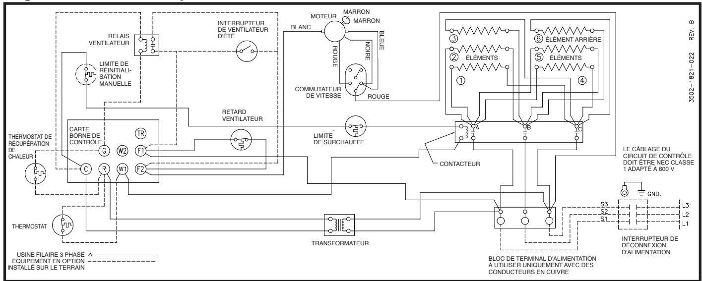
Diagramme 6: 6 éléments, 6 phases (des modèles 3END3 et 2YU78)
