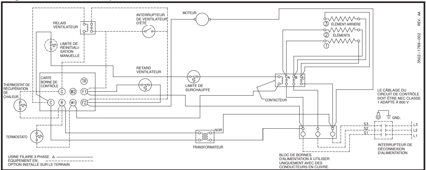
Diagramme 2: 3 éléments, 3 phases (des modèles 2YU59 et 2YU70)
