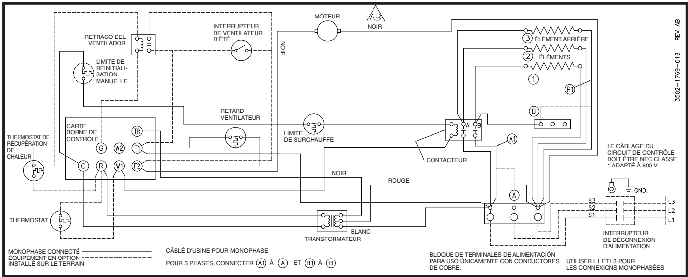
Diagramme 12: 3 éléments, monophasé et triphasé (modèle 2YU68)
