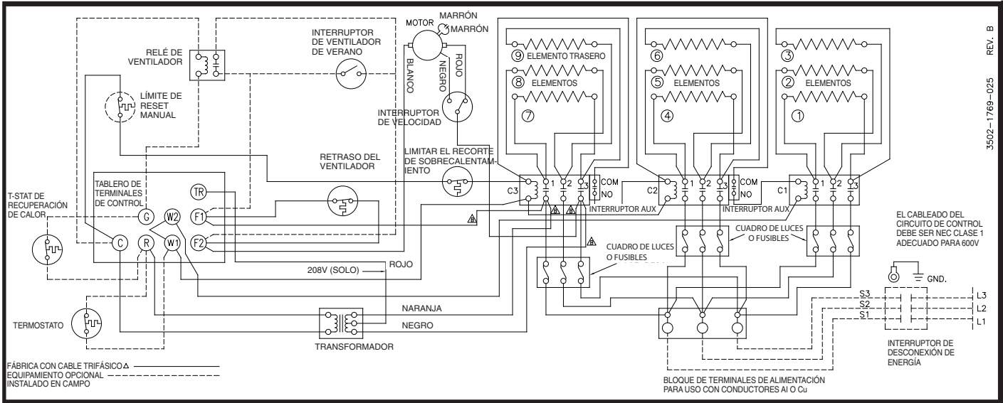
Diagrama 9: 9 elementos, 3 contactores, trifásico
