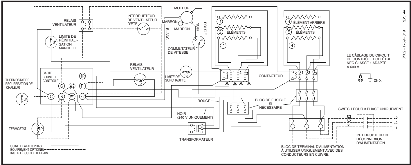
Diagramme 13: 6 éléments, 2 contacteurs, triphasés (modèle 2YU79)
