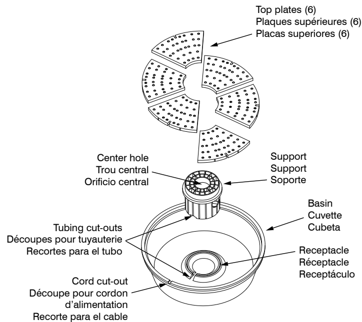
Fig. 2 - DFB36
