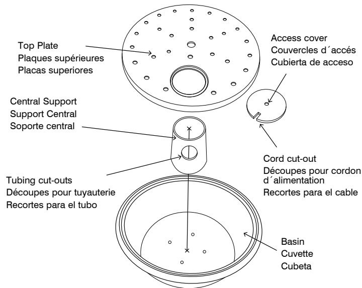
Fig. 1 - DFB30
