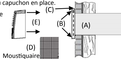
VUE LATÉRALE du couvercle du capuchon
