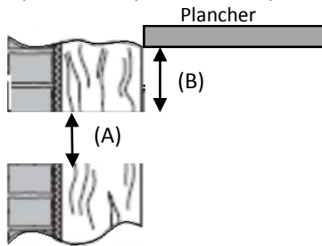
VUE LATÉRALE du mur extérieur
