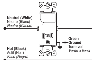
Wiring Diagram Schema de câblage Diagrama de Alámbrado
