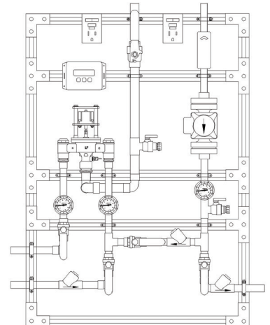
PNV-100-LF Proton Megatron
