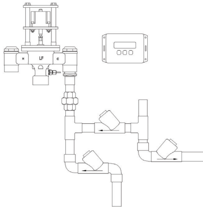
PNV-125-LF-R Simple Recirculation
