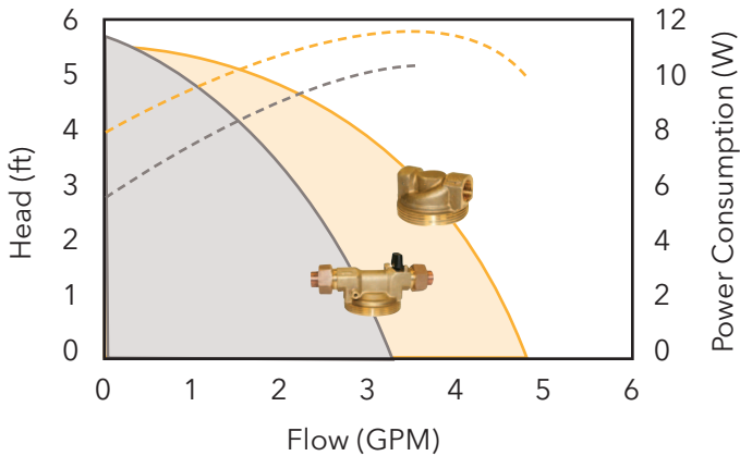
E1 Pump Curves
