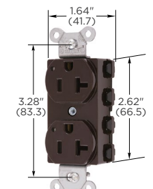
SNAP5362L
