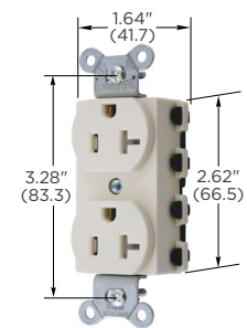
SNAP5362LATRA
