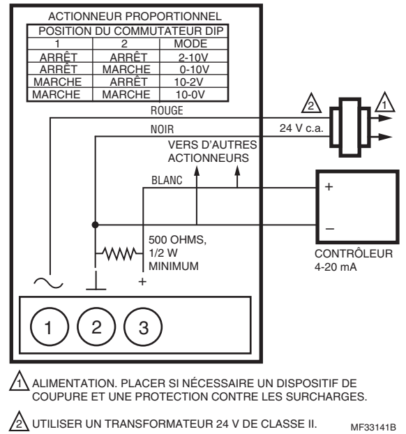
Fig. 19. MVN713 avec régulateur 4-20mA.
