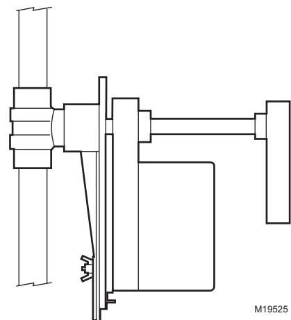
Fig. 4. Installation verticale du clapet.
