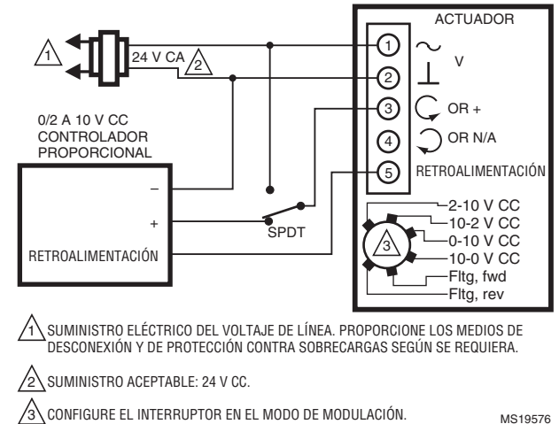
Fig. 12. MS7505 con control de sobrecomando para la posición completamente abierta (configuración del modo de modulación).
