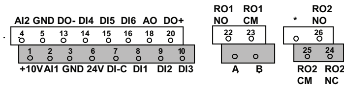
Fig. 24. Bornes de raccordement de commande du SmartVFD Compact.
