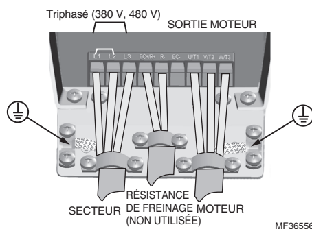
Fig. 16. Raccordements électriques du SmartVFD HVAC2, MI4.
