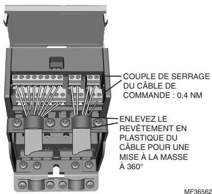
Fig. 22. Installation des câbles de commande. MI1 - MI3.
