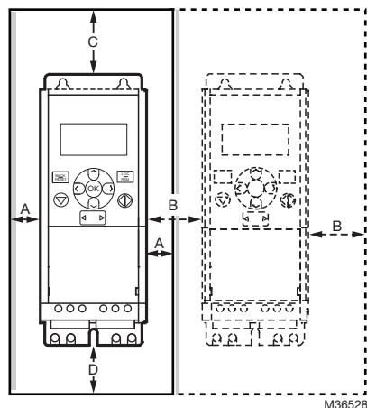
Fig. 13. Espace d'installation.
