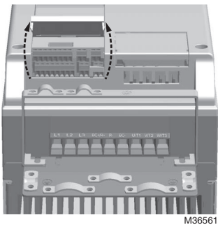
Fig. 21. Open the lid, MI4 - MI5.
