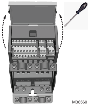
Fig. 20. Open the lid, MI1 - MI3.
