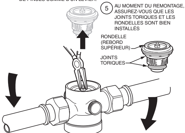
Fig. 4. Remplacement de la cartouche FK06.
