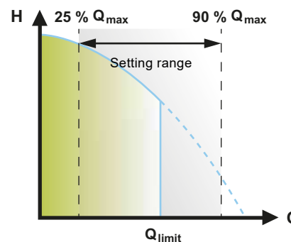
Fig. 28 FLOW_{LIMIT}
