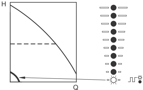
Fig. 18 Min. curve duty
