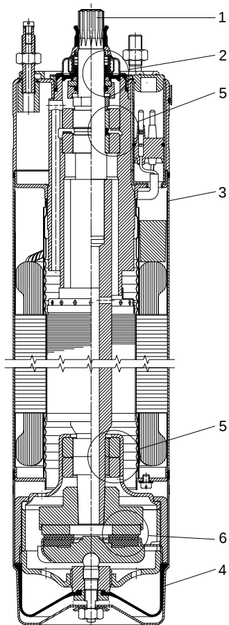
Fig. 18 MS 4000 motor
