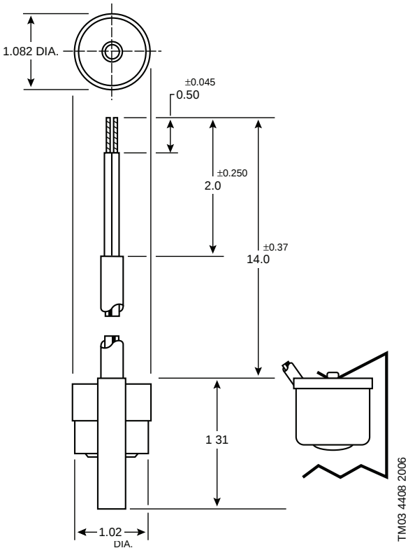
Fig. 4 AquaStat dimensions
