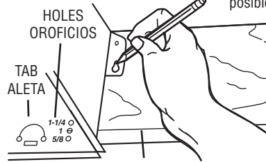
BOTTOM EDGE OF JOIST BORDE INFERIOR DE LA VIGUETA
