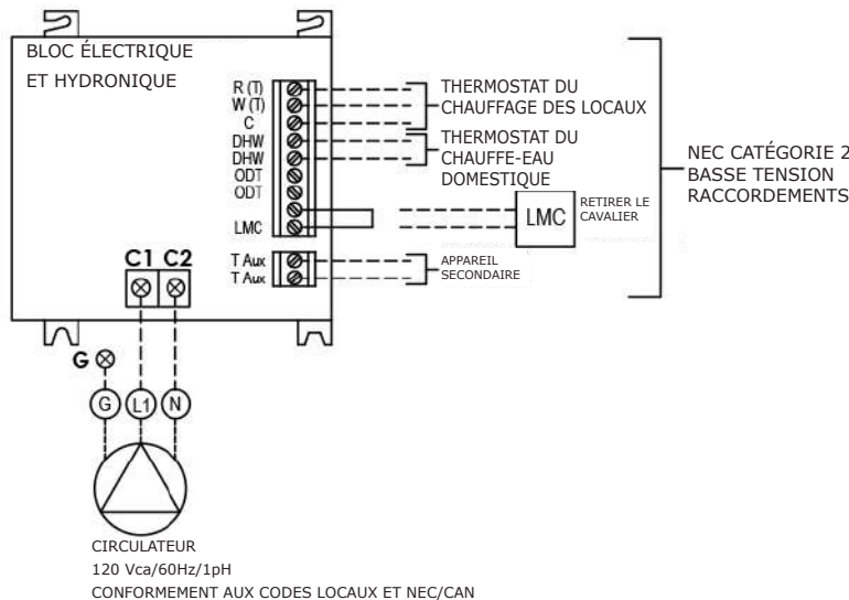
Figure 6 - Raccordement du thermostat et du circulateur
