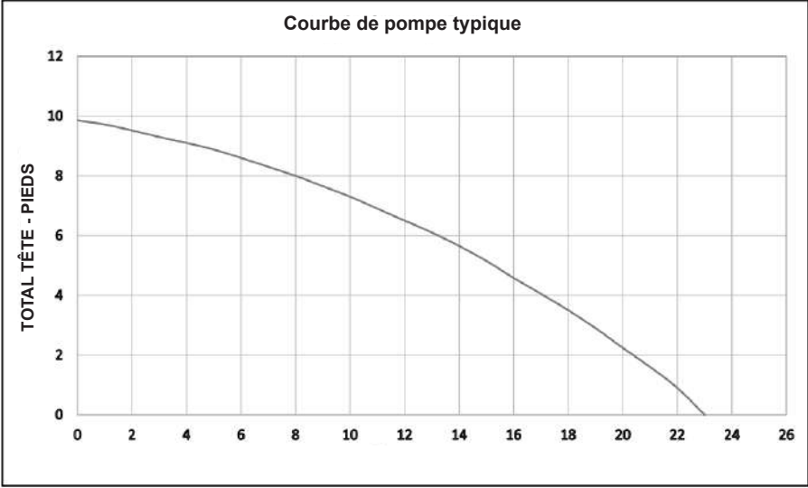
Figure 1B - Courbe typique de la pompe
