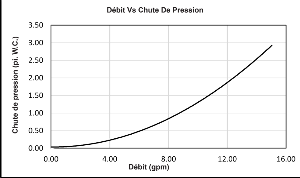
Figure 1C : chute de pression de la chaudière
