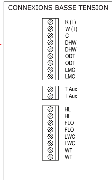
Figure 8 - Câblage basse tension du panneau de contrôle Board
