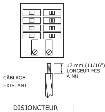
Figure 5 - Schéma de câblage
