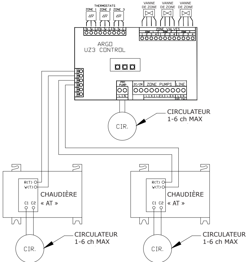
Figure 13 - Trois zones avec soupapes de régulation par zone – 2 chaudières
