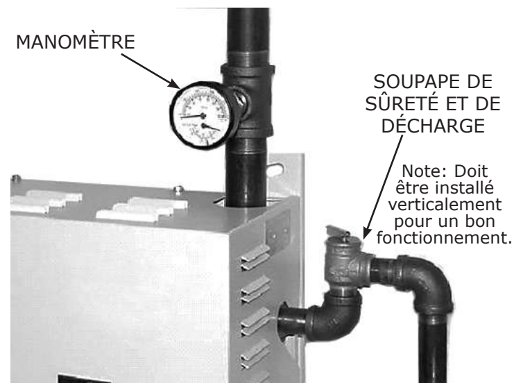
Figure 1A - Soupape de sûreté et de décharge
