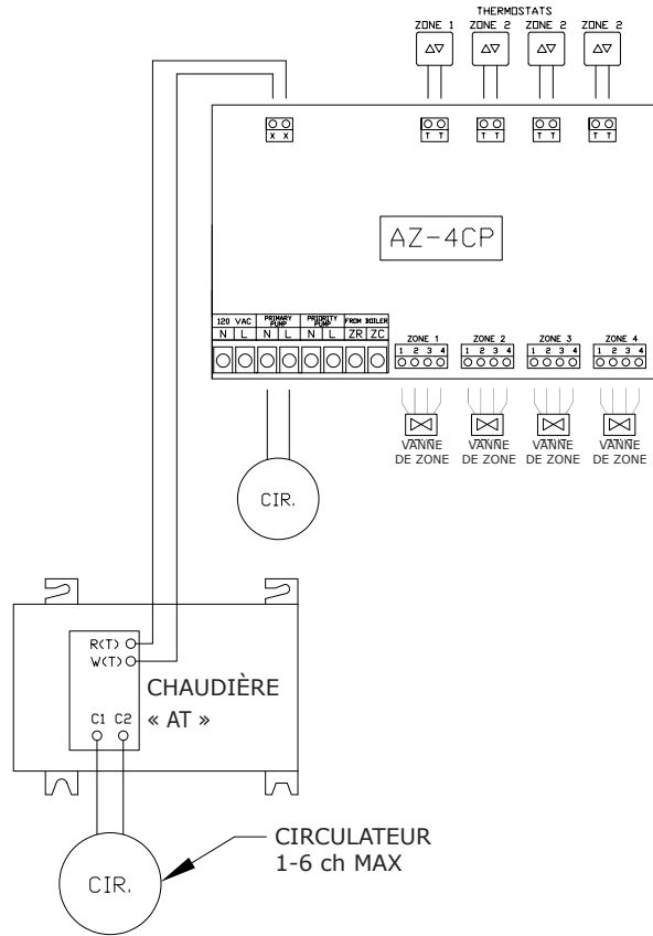
Figure 15 - Trois zones avec circulateurs
