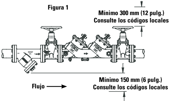
INSTALACIÓN HORIZONTAL DEL MONTAJE DE RETENCIÓN DOBLE SERIES 850, LF850 Y DEL MDRD SERIES 856, 856ST (vista frontal, se muestra con filtro)
