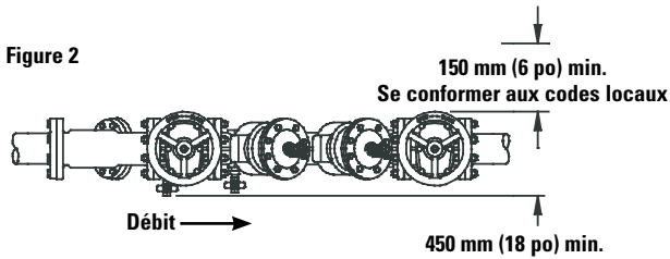
INSTALLATION HORIZONTALE DU DISPOSITIF À DOUBLE CLAPET DES SÉRIES 850 ET LF850 ET DU DÉTECTEUR À DOUBLE CLAPET DE SÉRIE 856 ET 856ST (Vue de dessus, illustrée avec une crépine)
