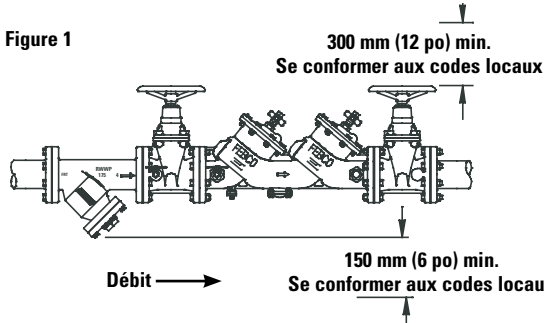
INSTALLATION HORIZONTALE DU DISPOSITIF À DOUBLE CLAPET DES SÉRIES 850 ET LF850 ET DU DÉTECTEUR À DOUBLE CLAPET DE SÉRIE 856 ET 856ST (Vue de face, illustrée avec une crépine)
