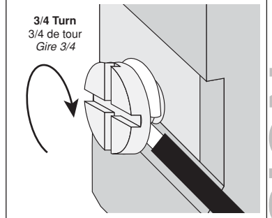
Fig. 2 Side Wire / Câblage Latéral / Cableado Lateral
