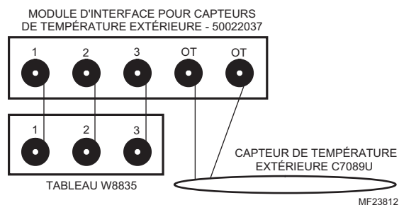
Fig. 1. Schéma de raccordement du module d'interface pour capteurs de température extérieure.
