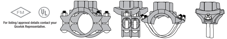
Fig. 7045 (U-Bolt)
