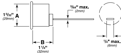
Rim 3216
