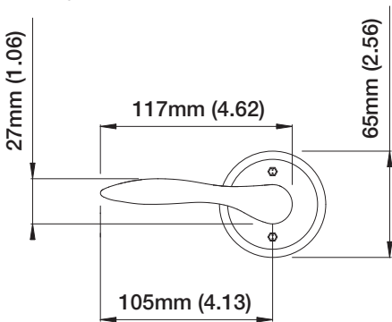
Passage Set LH Shown
