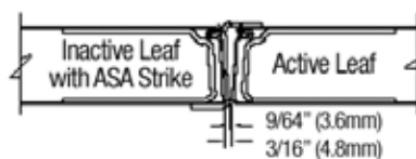
Z Astragal
