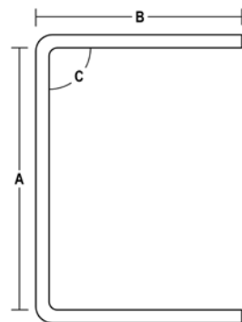
K41 90° SURFACE EDGE GUARD
