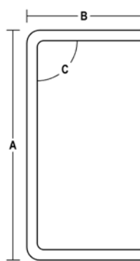
K37 90° MORTISE EDGE GUARD
