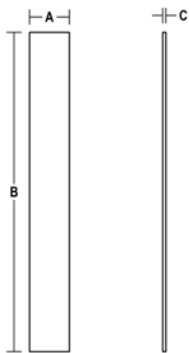
K35 1.5" ASTRAGAL
