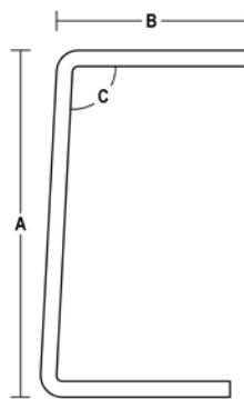
K38 93° MORTISE EDGE GUARD
