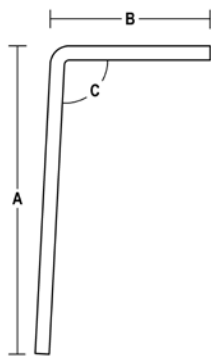
K40 93° MORTISE EDGE GUARD - HALF
