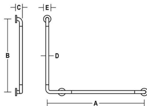
G241-70-P 40" X 30" X 90° X GRAB BAR - Ø 1-1/4"
