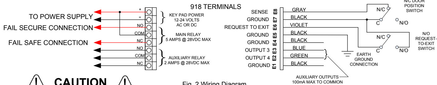
Fig. 2 Wiring Diagram
