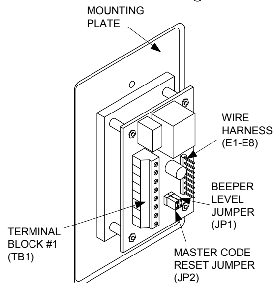
Fig. 1 Keypad
