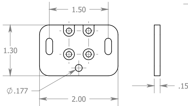
OPTIONAL MOUNT PLATE PN: 1156
