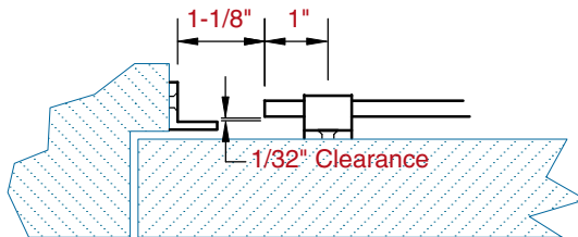
L STRIKE: Out Swinging Door
