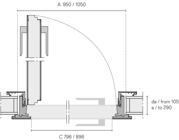
A. Luce netta falso telaio Subframe dimension C. Luce netta passaggio Opening dimension
