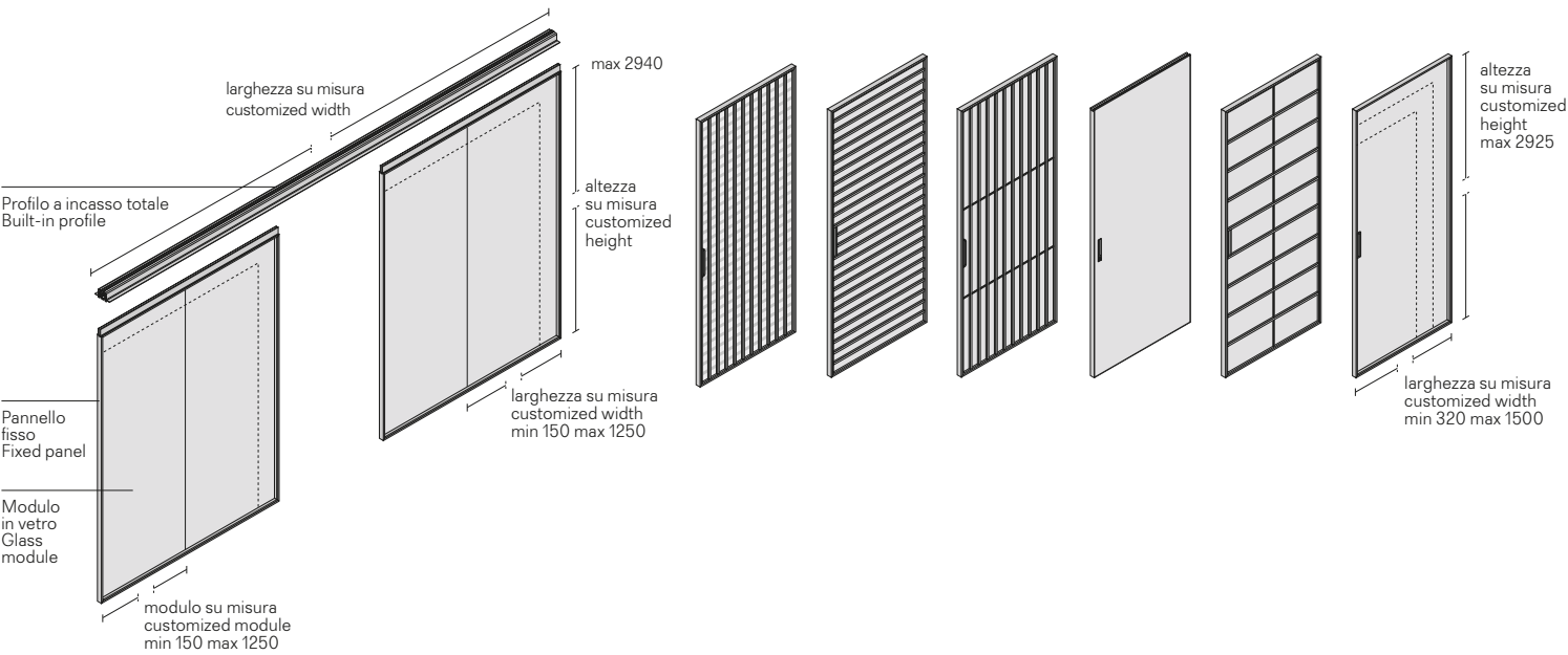
Dimensioni sistema interparete Spazio e porte abbinate Spazio partition wall system dimension and combined doors
