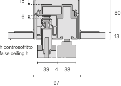
Profilo doppio incasso totale Double built in profile
