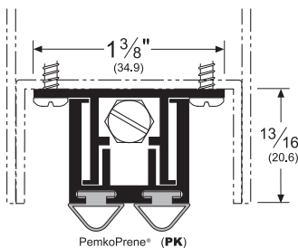
PemkoPrene (PK)
