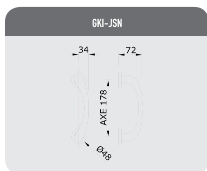
Maniglione axe mm178 con rosetta Nika Pull Handle axe mm178 on Nika rose
