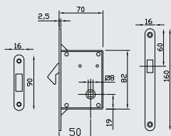
Serratura csv per porte scorrevoli: Quadro 8mm - entrata 50mm Square 8mm: - backset 50mm
