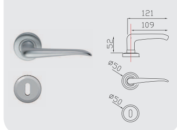
Maniglia con rosetta/bocchetta Artax Lever on Artax rose and key hole
