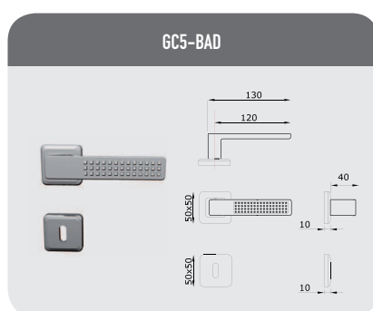
Maniglia con rosetta/bocchetta Qbe Lever on Qbe rose and key hole
