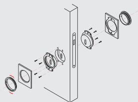
Coppia placca incasso con foro chiave Set flush plate with standard key hole n. 1 set
