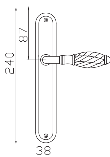
cod. GCW-AAS Maniglia con placca Astra Lever on Astra plate
