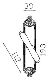
cod. GLA-LAH Lara cremonese con placca Heide Lara cremon on Heide plate ■ n. 2 pz
