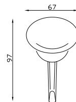
Cod. G6D-430 GRA-4153 Portabito GRA-4153 Coat hook n. 2 pz
