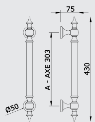
Maniglione axe mm303 Pull Handle axe mm303 n.1 pz
