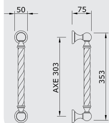
Maniglione axe mm303 Pull Handle axe mm303 n.1 pz
