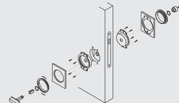
Coppia placca incasso con nottolino Set flush plate with turn and release n. 1 set
