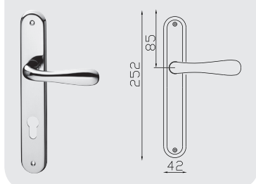
Maniglia con placca Thalassia Lever on Thalassia plate
