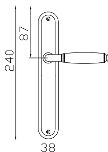
cod. eb. GSB-AAS cod. pal. GSP-AAS Maniglia con placca Astra Lever on Astra plate
