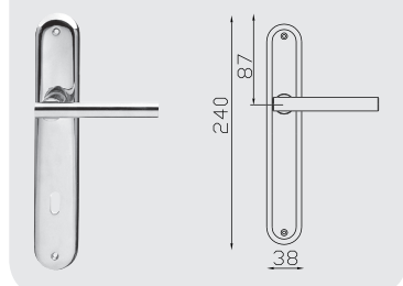
Maniglia con placca Astra Lever on Astra plate
