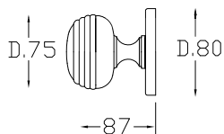
cod. GEL-FAI Pomolo fisso "A" singolo Knob "A" single fixed n. 1 pz
