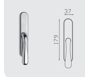
Cremonese/Martellina con placca Thalassia C.V. Movimento non incluso nel prezzo Cremon/Martellina on Thalassia screw cover plate Price of mechanism not included
