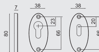
Historia Ov. paia Bocchette FC/Yale Historia Ov. pair key hole PK/Yale
