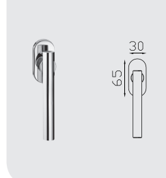
Maniglia con Dreh-Kipp Nika Lever on Nika Dreh-Kipp
