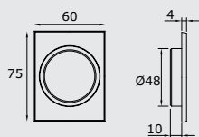
Xbe Uno placca incasso Xbe Uno flush plate
