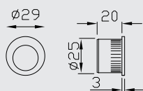
Onda trascinatore frontale Onda pull ring
