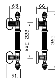
cod. G1B-QUB Maniglione tipo "B" singolo Pull handle type "B" single n. 1 pz
