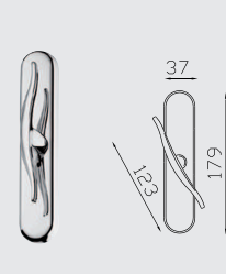
Onda cremonese/Martellina con placca Thalassia C.V. Movimento non incluso nel prezzo Onda cremon/Martellina on Thalassia screw cover plate Price of mechanism not included n. 2 pz
