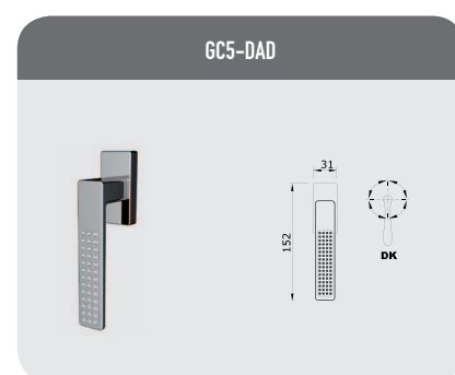
Maniglia con Dreh-Kipp Qbe Lever on Qbe Dreh-Kipp
