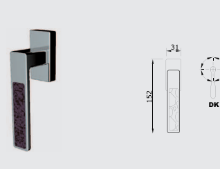
Maniglia con Dreh-Kipp Qbe Lever on Qbe Dreh-Kipp
