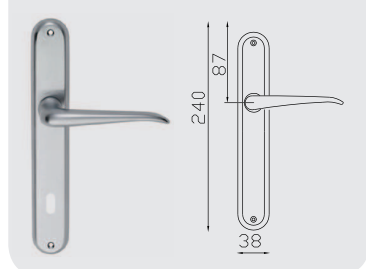
Maniglia con placca Astra Lever on Astra plate
