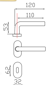
cod. GLE-BAY Maniglia con rosetta/bocchetta OP ovale Lever on OP ovale rose and key hole ■ n. 1 set
