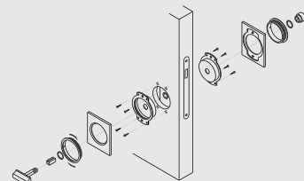
Coppia placca incasso con nottolino Set flush plate with turn and release n. 1 set
