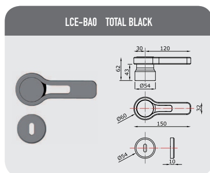
Maniglia con rosetta/bocchetta Core Lever on Core rose and key hole
