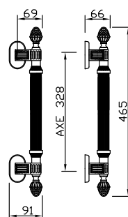
cod. G1B-QUA Maniglione tipo "A" singolo Pull handle type "A" single n. 1 pz
