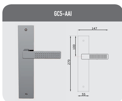
Maniglia con placca Libra Lever on libra plate
