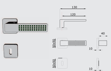
Maniglia con rosetta/bocchetta Qbe Lever on Qbe rose and key hole
