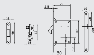
Serratura csv per porte scorrevoli: foro chiave - entrata 50mm Locks for sliding door: key hole - backset 50mm
