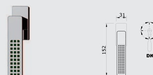
Maniglia con Dreh-Kipp Qbe Lever on Qbe Dreh-Kipp
