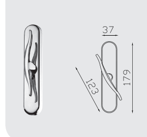
Onda cremonese/Martellina con placca Thalassia C.V. Movimento non incluso nel prezzo Onda cremon/Martellina on Thalassia screw cover plate Price of mechanism not included
