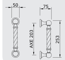
Maniglione axe mm203 Pull Handle axe mm203 n.1 pz
