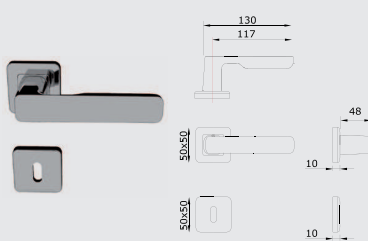
Maniglia con rosetta/bocchetta Qbe Lever on Qbe rose and key hole
