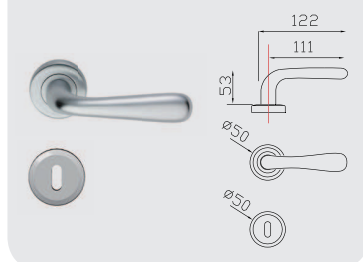
Maniglia con rosetta/bocchetta Artax Lever on Artax rose and key hole
