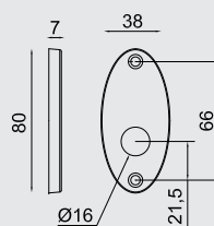
Historia Ov. Paia Rosette Historia Ov. Pair roses
