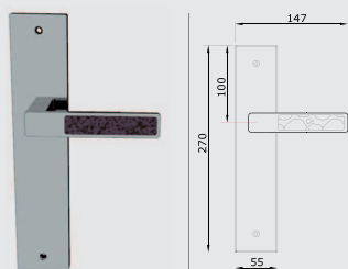
Maniglia con placca Libra Lever on libra plate
