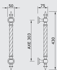
Maniglione axe mm303 Pull Handle axe mm303 n.1 pz
