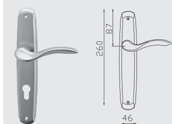
Maniglia con placca Asia Lever on Asia plate
