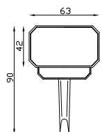
Cod. G6D-220 GRA-202 Portabito GRA-202 Coat hook n. 2 pz
