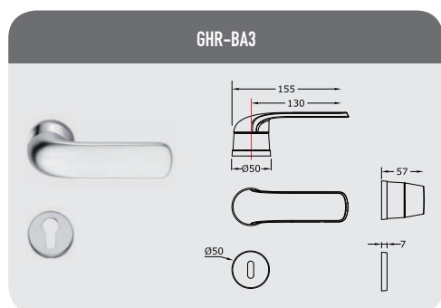
Maniglia con rosetta/bocchetta Lever on rose and key hole
