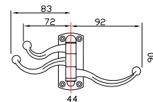
Cod. G6D-250 GRA-215 Portabito GRA-215 Coat hook n. 6 pz
