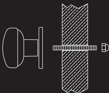
MONTAGGIO POMOLO SINGOLO FISSO TIPO A/B CON VITE PASSANTE MOUNTING FOR FIXED KNOB A/B THROUGH SCREW
