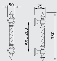
Maniglione axe mm203 Pull Handle axe mm203 n.1 pz
