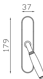
cod. eb. GSB-LMT - cod. pal. GSP-LMT Cremonese/Martellina con placca Thalassia C.V Movimento non incluso nel prezzo Cremon/Martellina on Thalassia C.V screw cover plate Mechanism not included in the price
