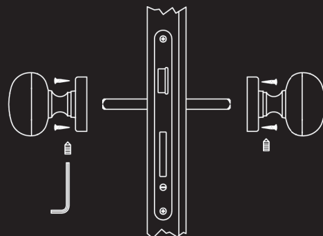
MONTAGGIO POMOLI ACCOPPIATI GIREVOLI TIPO B MOUNTING FOR KNOBSET B
