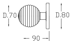
cod. GEY-FAI Pomolo fisso "A" singolo Knob "A" single fixed n. 1 pz
