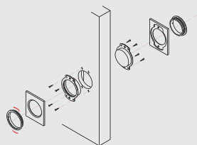
Coppia placca incasso cieca Set flush plate blind n. 1 set
