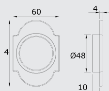
Xbe Tre placca incasso Xbe Tre flush plate
