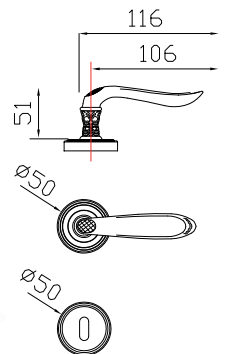
cod. GCR-BAG Maniglia con rosetta/bocchetta Gaia Lever on Gaia rose and key hole ■ n. 1 set
