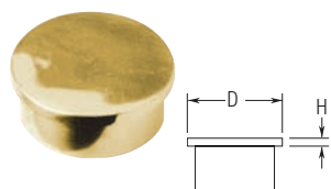
600 Flush End Cap
