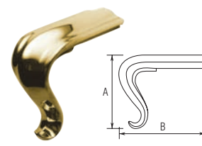
H1600LT Cap Rail Lamb Tongue End
