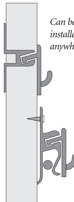
P3 Roller Clip
