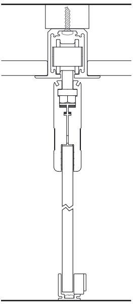
RECESSED / EMPOTRADO TOP TRACK / PERFIL TOP
