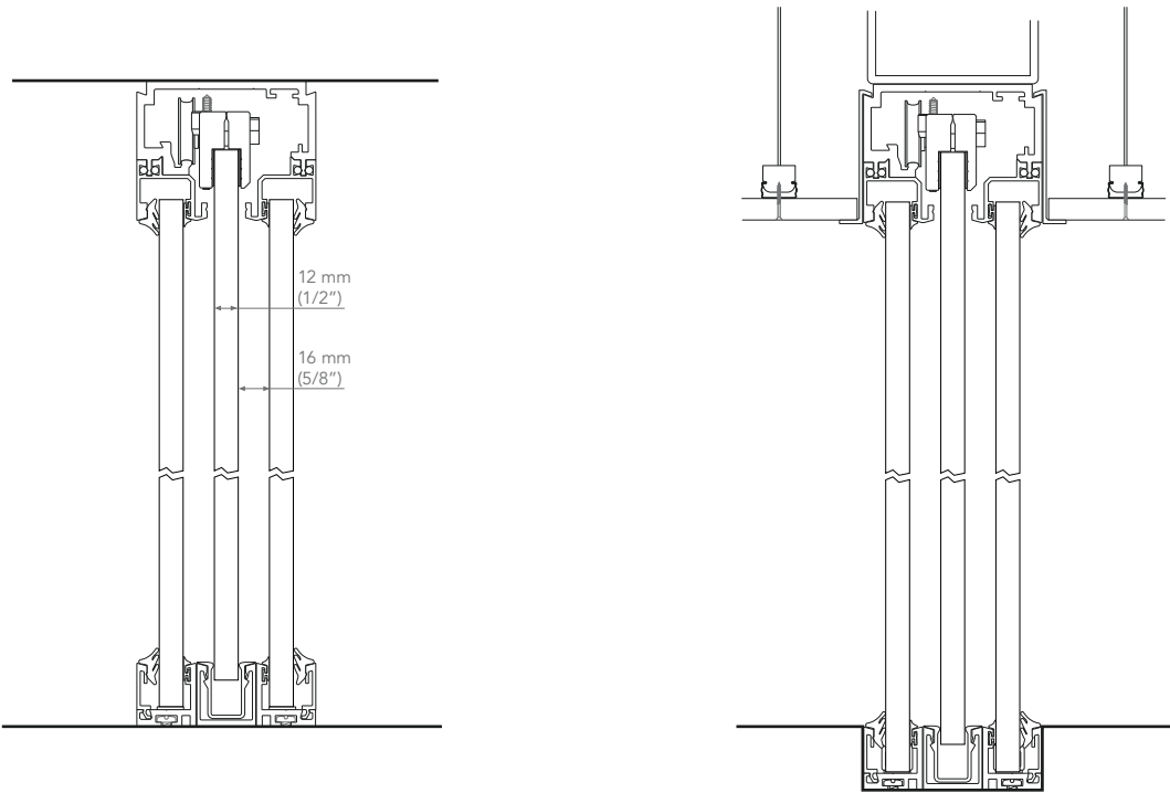
DOUBLE FIXED GLAZING / DOBLE VIDRIO FIJO
