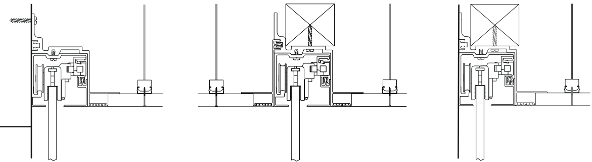
WITH LINTEL / CON DINTEL
