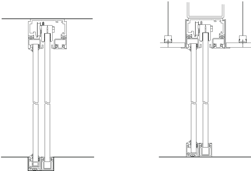
SINGLE FIXED GLAZING / UN VIDRIO FIJO
