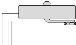
Top Jamb
