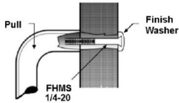
Standard Thru Bolt - .E
