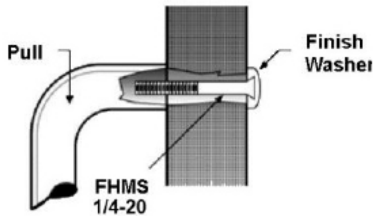
Standard Thru Bolt - .E
