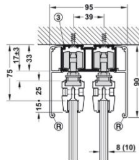
Deckenmontage mit Doppellaufschiene und Clipblende 90 mm
