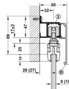
Wandmontage mit Laufschiene und Clipblende 90 mm
