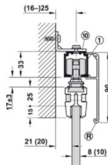
Wandmontage mit Montagewinkel und Clipblende 90 mm
