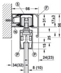
Wandmontage mit Laufschiene und Clipblende 56 mm sowie Clipblende auf dem Glasklemmschuh
