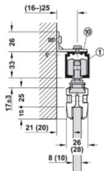
Wandmontage mit Montagewinkel
