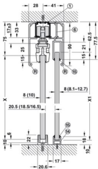
Deckenmontage mit Laufschiene und Clipblende 90 mm inkl. Festteil. Bei Glasdicke 10 mm Dichtung einseitig, bei Glasdicke 8–12,7 mm nassversiegeln
