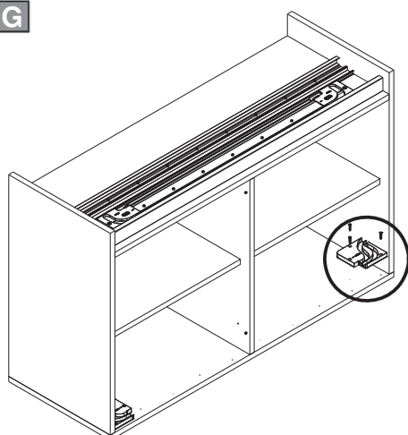
Aufgesetzte Führung Surface-mounted guide Guidage en applique
