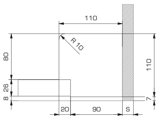
Optionale Einbauvariante mit versenkter Führung (Kleben) Optional mounting example with inset guide (Glue) Variante de montage optionnelle avec guidage encastré (Coller)
