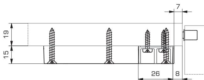
Aufgesetzte Führung Surface-mounted guide Guidage en applique
