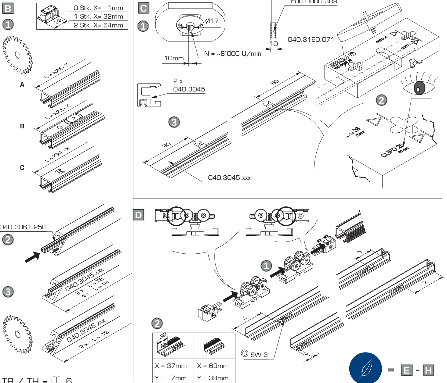
Befestigungsvarianten A - C / Mounting options A - C / Variantes de fixation A - C: 4
