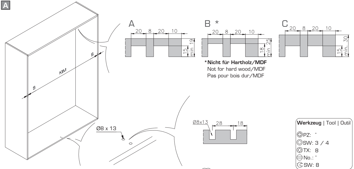
Befestigungsvarianten A - C / Mounting options A - C / Variantes de fixation A - C: 4
