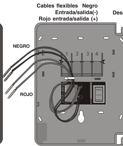
Cables Flexibles de la BG-12 de Acción Singular
