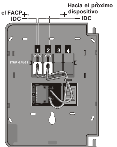
Alambrado de la BG-12, 12L, 12LSP de Acción Doble
