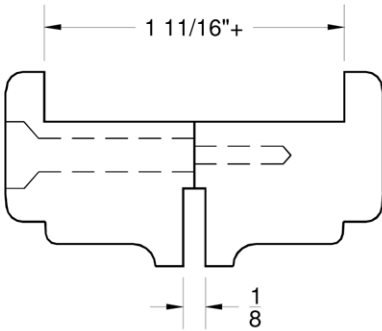
1 3/4" DOORLITE MLDG
