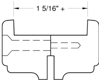
1 3/8" DOORLITE MLDG
